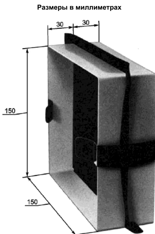
Рисунок А.1 - Монтажная рамка для вертикального индикатора
