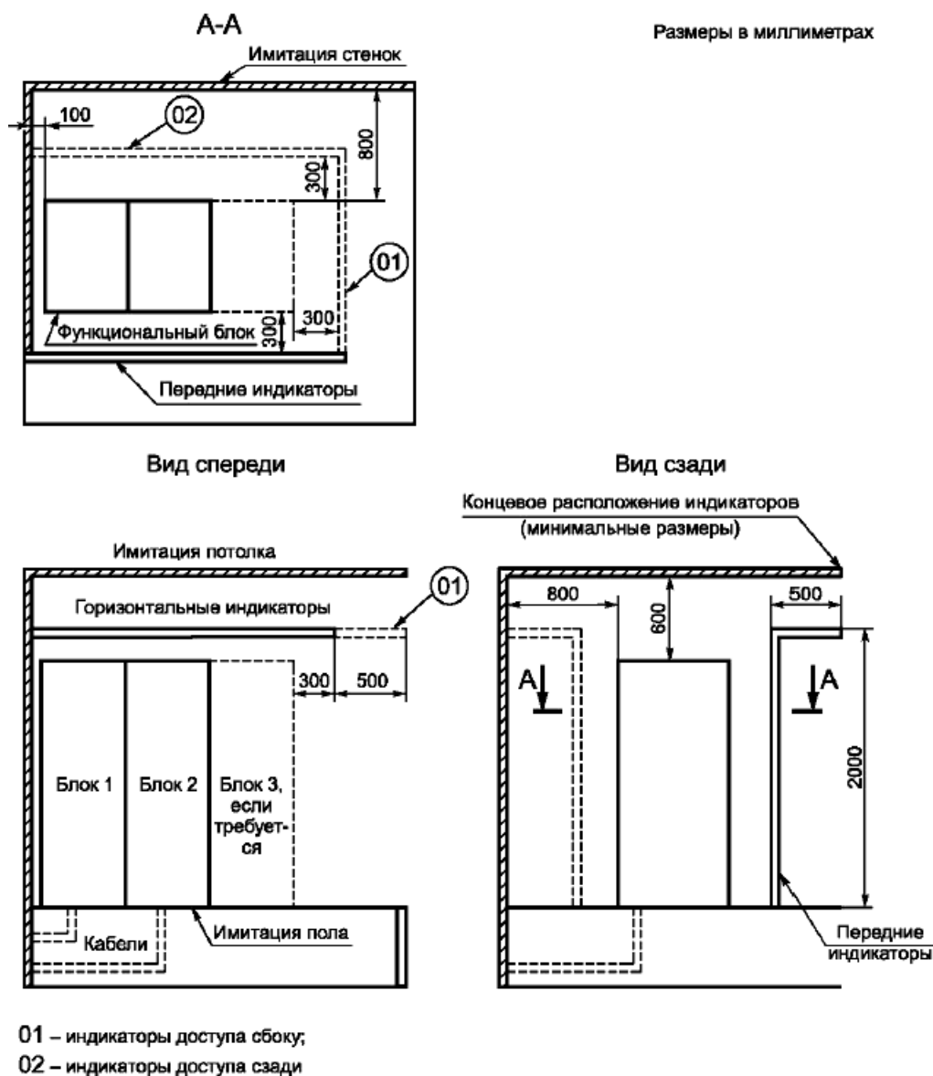
Рисунок А.4 - Имитация помещения и положение индикаторов для типа доступа А, высота функционального блока 1,5 м и выше
