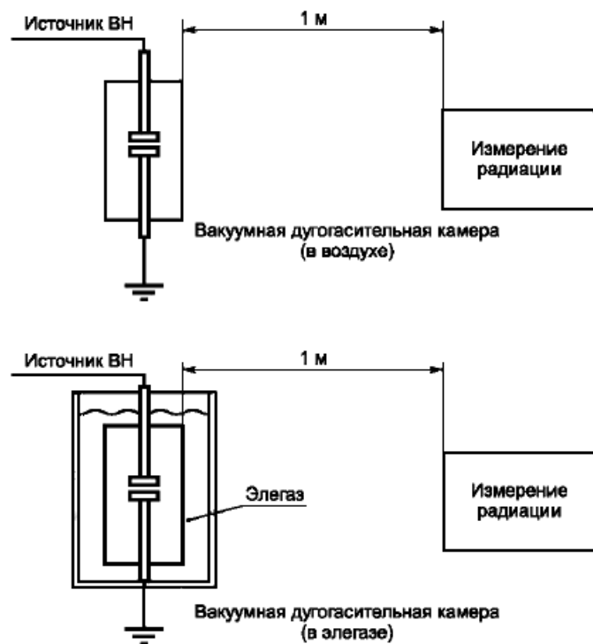
Рисунок 2 - Место монтажа дозиметра
