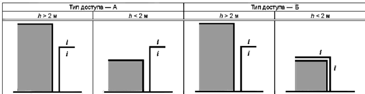
Рисунок А.2 - Горизонтальный индикатор
