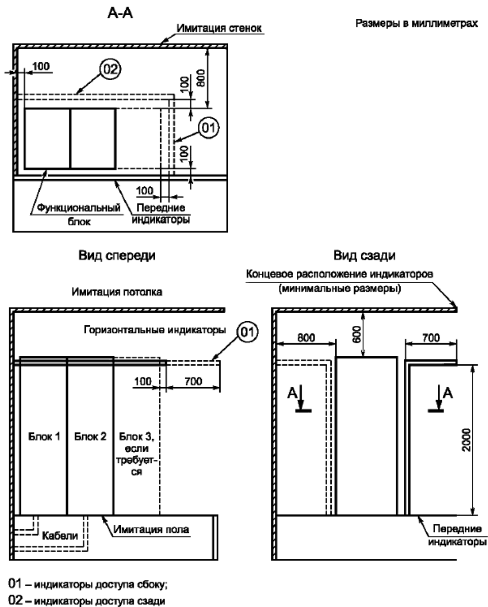
Рисунок А.5 - Имитация помещения и положение индикатора для типа доступа В, высота функционального блока 2,0 м и выше
